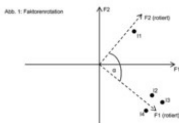
Abb. 1 Faktorenrotation
