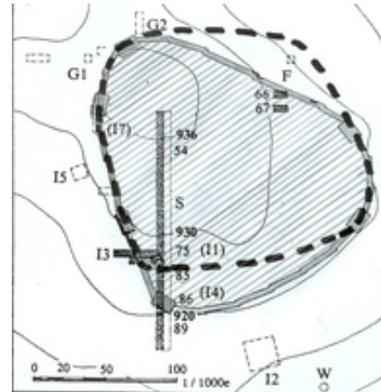
Abb. 10 Plan von Gebel er-Rumēde (schraffiert: Stadtanlage der Mittelbronzezeit, gestrichelte Linie: erschlossene Ausdehnung der Siedlung des 11./10. Jh.s v. Chr.).
