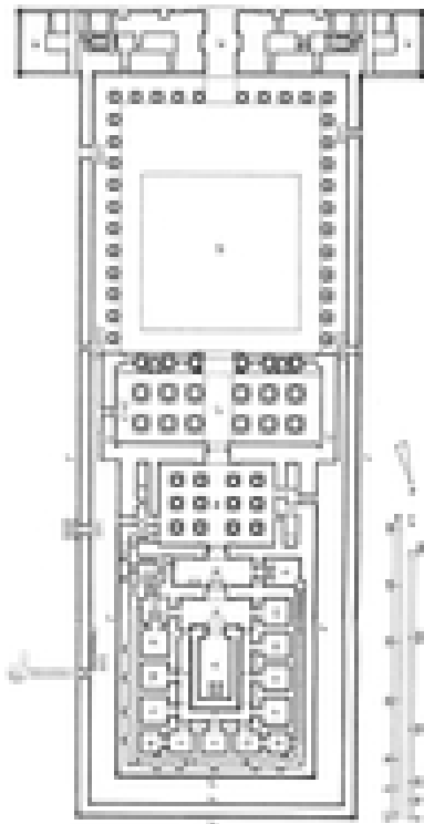
Abb. 3 Grundriss des Tempels von Edfu (im Artikel verweisen Großbuchstaben in runden Klammern auf diesen Grundriss).
